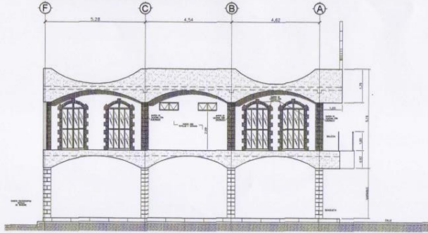
ELEVACIÓN LATERAL MUNICIPALIDAD DE SANSARÉ, EL PROGRESO
